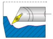
内孔车刀 Internal turning tool
