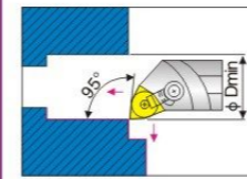
内孔车刀 Internal turning tool
